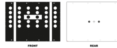
Kalibratiebord voor VW + MB Art.nr. WW01000670
