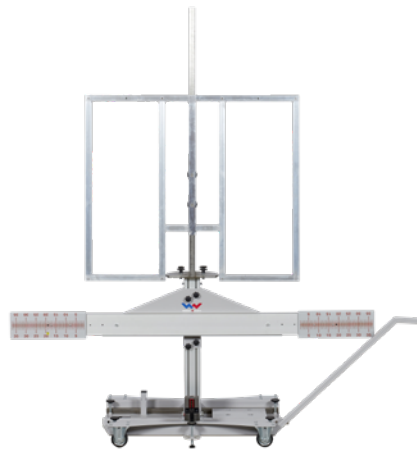
Uitbreiding camerakalibratie bestel- en personenwagens* Art.nr. WW01000663
