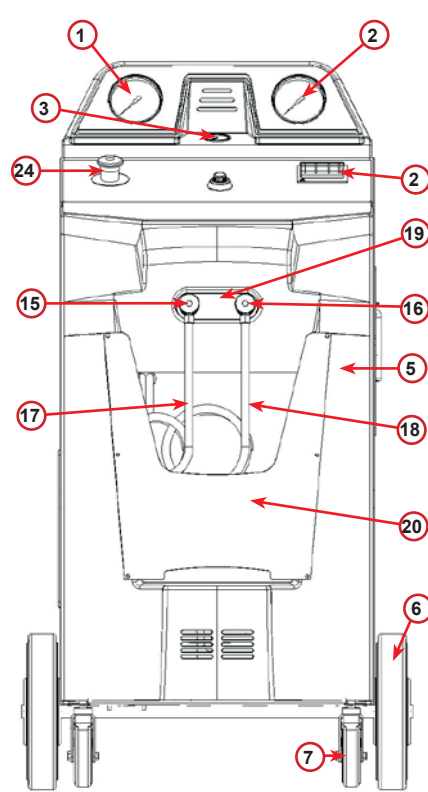
Abb. 002 Ansicht vorne
